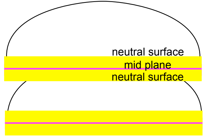
separate membranes
