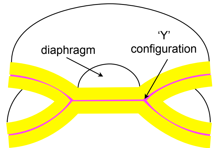
hemifusion
